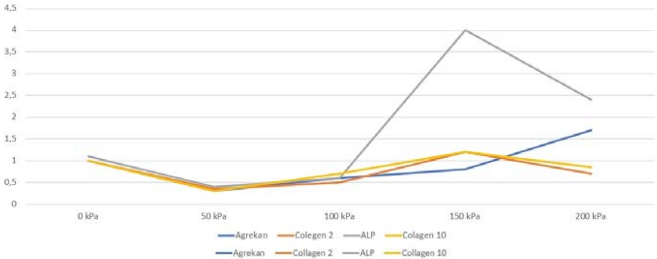
Rycina 3. Relatywna ekspresja mRNA przy różnych wartościach ciśnienia podczas badania in vitro. Figure 3. The relative mRNA expression at various pressure values during the in vitro test.
